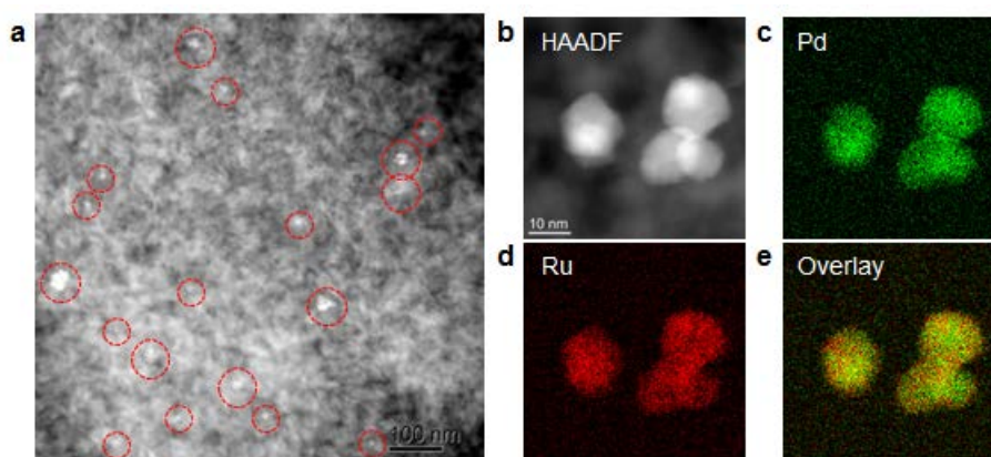
図1 高角散乱環状暗視野走査透過型電子顕微鏡（HAADF-STEM）による元素マッピング (a) HAADF-STEM イメージ赤い破線で囲まれた輝点が担持された PdRu-NPs (b) PdRu-NPs の拡大 HAADF イメージ (c) Pd の元素マッピング (d) Ru の元素マッピング (e) Pd と Ru の元素マッピングの重ねあわせ、ナノ粒子内に Pd と Ru が一様に分布しており、原子レベルで混合した固溶体ができていることが分かる。
