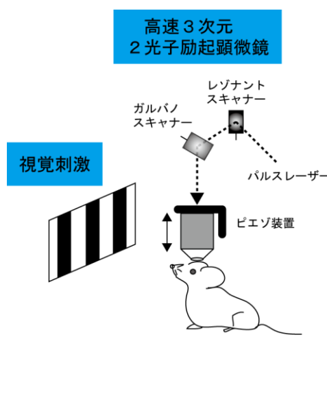
(図1) 高速3次元2光子励起顕微鏡。視覚刺激を与えたときの神経細胞の活動を、カルシウム指示薬を用いて3次元的に記録した。
