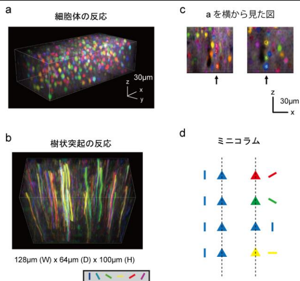
(図2) (a, b) 方位選択性について3次元高速カルシウムイメージングを細胞体(a)と樹状突起(b)に対して行い、方位選択性の3次元カラーマップを作成。(c) 細胞体の3次元カラーマップを横から2次元で見ると、方位選択性が縦1列に揃っている場合と揃っていない場合が見られた。(d) ミニコラムには、方位選択性が揃っているものと、揃っていないものがあった。詳細な解析の結果、全体の約3割のミニコラムで方位選択性が揃っていることが分かった。
