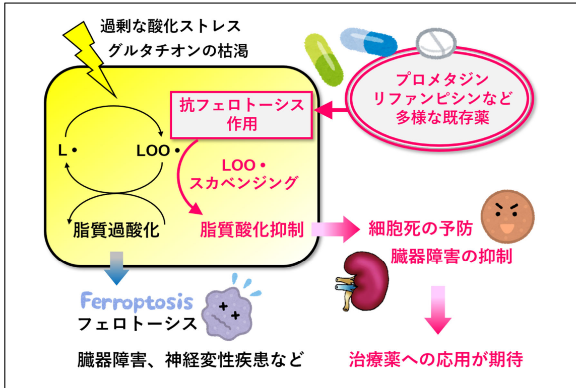
図 3. 既存薬がフェロトーシスを抑える仕組み LOO·, 脂質ペルオキシラジカル; L·, 脂質ラジカル
