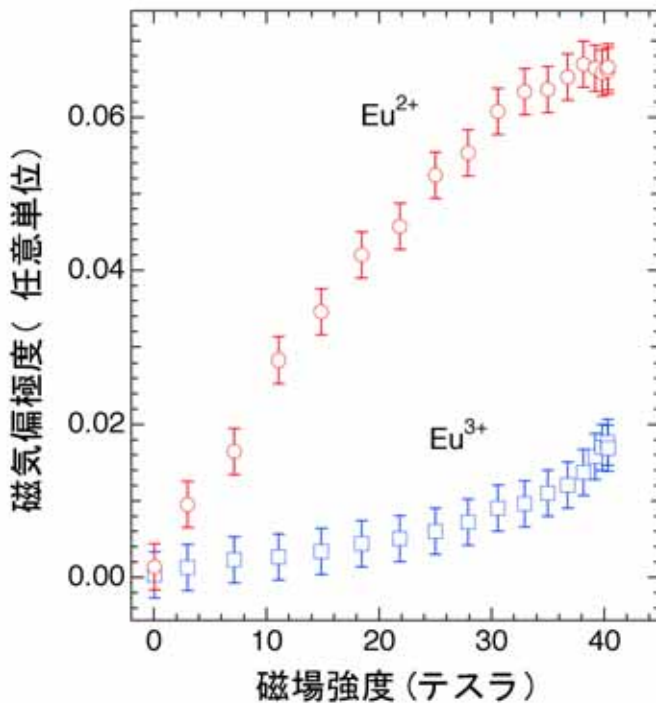
図4：ユーロピウム元素（Eu）の異なる電子価数状態（ \text{Eu}^{2+} 、 \text{Eu}^{3+} ）における磁気応答（磁気偏極度）の磁場依存性。2つの電子状態における磁気応答が全く異なる。これまではこの2つを区別することは不可能であったが今回の手法で可能になった。
