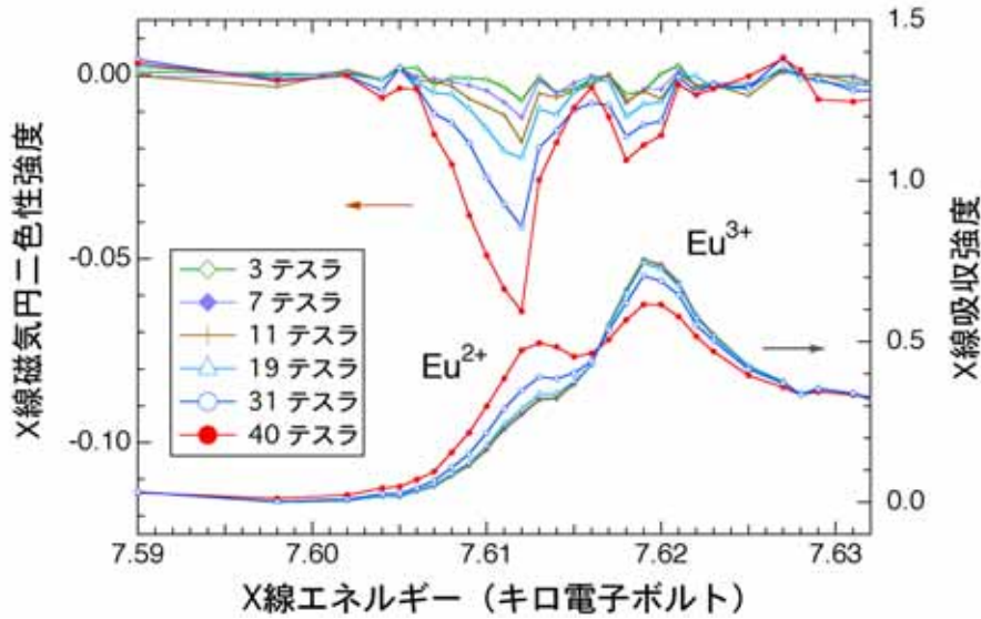
図3：ユーロピウム元素（Eu）のX線磁気円二色性（XMCD）スペクトル：[上]とX線吸収スペクトル：[下]の磁場依存性。2つの異なる電子状態 \text{Eu}^{2+} と \text{Eu}^{3+} が分離して観測されている。
