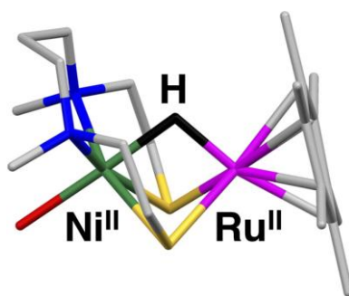
図1 燃料電池の電極触媒として用いたニッケルルテニウム分子触媒（小江触媒）
