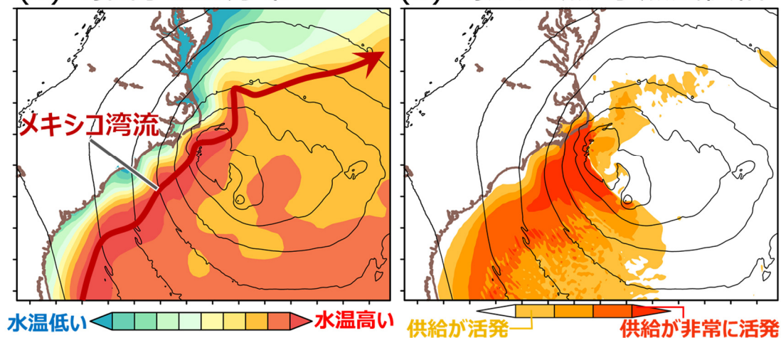
図 2. 低気圧が最も急発達した時刻（協定世界時 2018 年 1 月 4 日 6 時）の海面水温と海から大気への熱・水蒸気供給量の分布。地上における気圧も示している。
