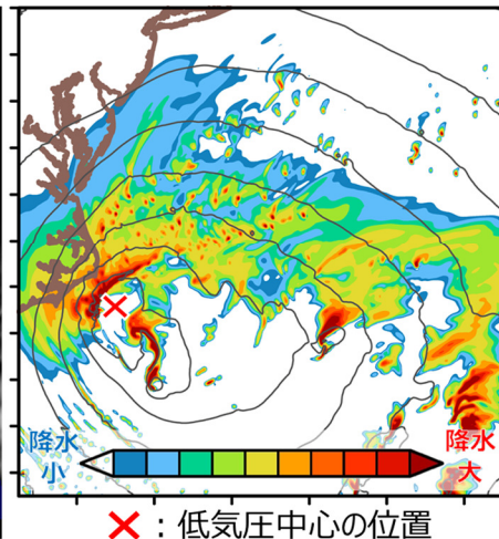
図1. 高解像度の数値シミュレーションで再現された「スーパー爆弾低気圧」に伴う雲の三次元構造と地上における降水と気圧の分布。時刻は低気圧が最も急発達した時刻（協定世界時2018年1月4日6時）。
