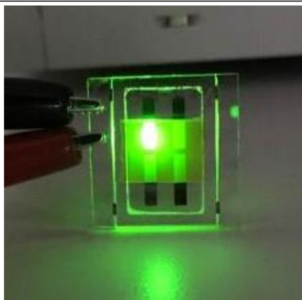
本研究で開発した明るく発光するペロブスカイトLED
