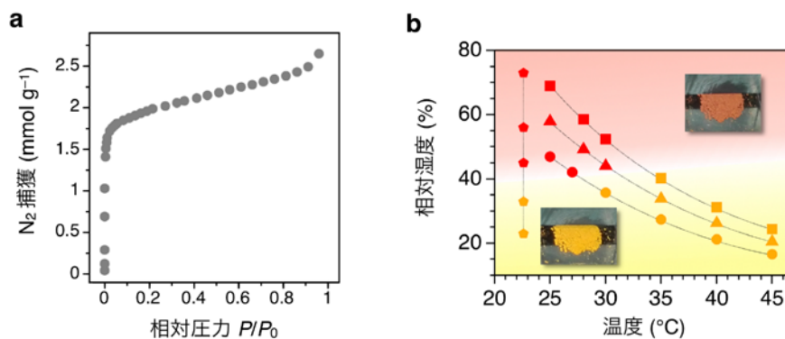
図 2 (a) -196 °Cにおける VPC-1 の窒素ガス吸着等温線。(b) 多孔質結晶 VPC-1 の発色に関する相対湿度-温度相図。●、▲、■ : 25 °Cにおける相対湿度 47, 58, 67%の状態から湿度を制御せずに温度を変化させたときの VPC-1 の色変化。五角形 : 温度一定 (22.6 °C) 条件で相対湿度を変化させたときの VPC-1 の色変化。内挿写真は赤色および黄色の状態の VPC-1 粉末の写真。
