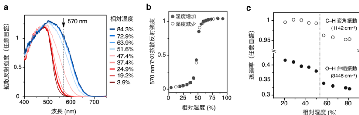
図3 (a, b) VPC-1 粉末の拡散反射スペクトル(a)および波長 570 nm における拡散反射強度 (b) の湿度依存性。(c) VPC-1 粉末の FT-IR スペクトルにおける C-H 変角振動 (○ : 1142\text{ cm}^{-1} ) および O-H 伸縮振動 (● : 3448\text{ cm}^{-1} ) の湿度依存性。
