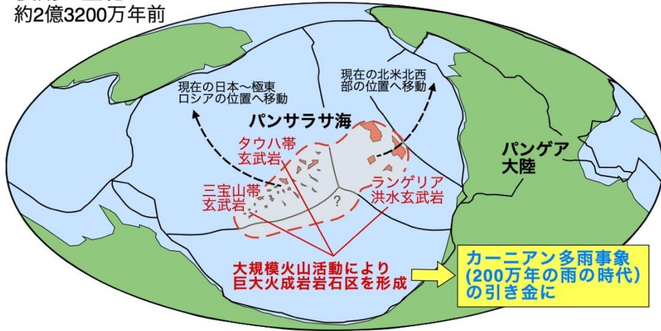
図1 後期三畳紀カーニアン地球の姿。超海洋パンサラサ海において大規模な火山活動が起こり、これが引き金となりカーニアン多雨事象が誘発された。このとき噴出した大量の玄武岩の岩体は、海洋プレート移動により分裂し、現在は日本、極東ロシア、北米北西部などに分布している。
