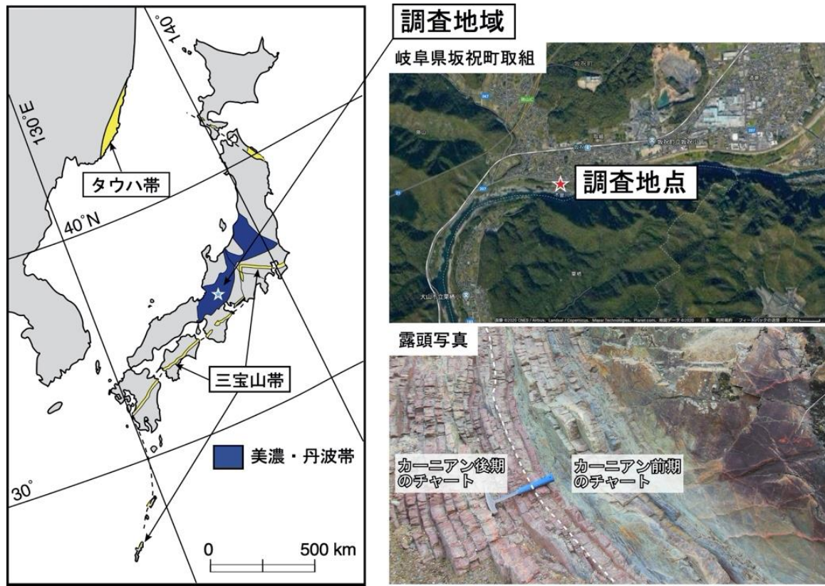
図3 カーニアンの大規模火山活動の証拠が発見された地域（岐阜県坂祝町取組）。研究対象は木曽川右岸に露出したチャートという岩石。
