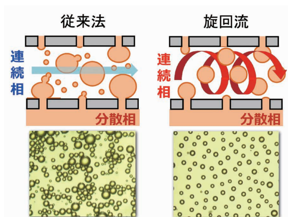
従来法による乳化と高速旋回流による乳化の比較。従来法では様々なサイズの液滴ができてしまっているが、旋回流方式ではほぼ均一なサイズの液滴になっている。
