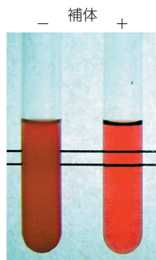
異種赤血球を補体が破壊すると、ヘモグロビンが放出されて赤血球細胞が消え、透明になってしまいます。
