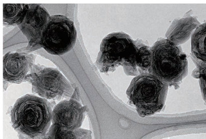
土壌のナノ粒子（粘土鉱物）
