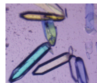
酵素の結晶
