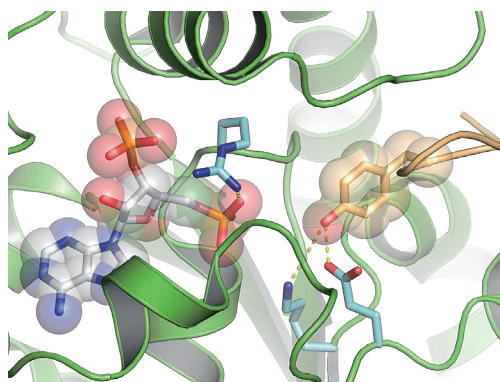
酵素の結晶
