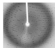
X線回折データ
