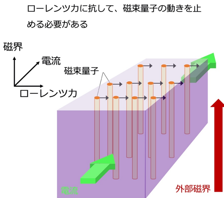
図 1: 外部磁界を印加すると量子化された磁束が超伝導体内に侵入する。この状態で電流を流すと磁束量子にはローレンツ力が働く。
