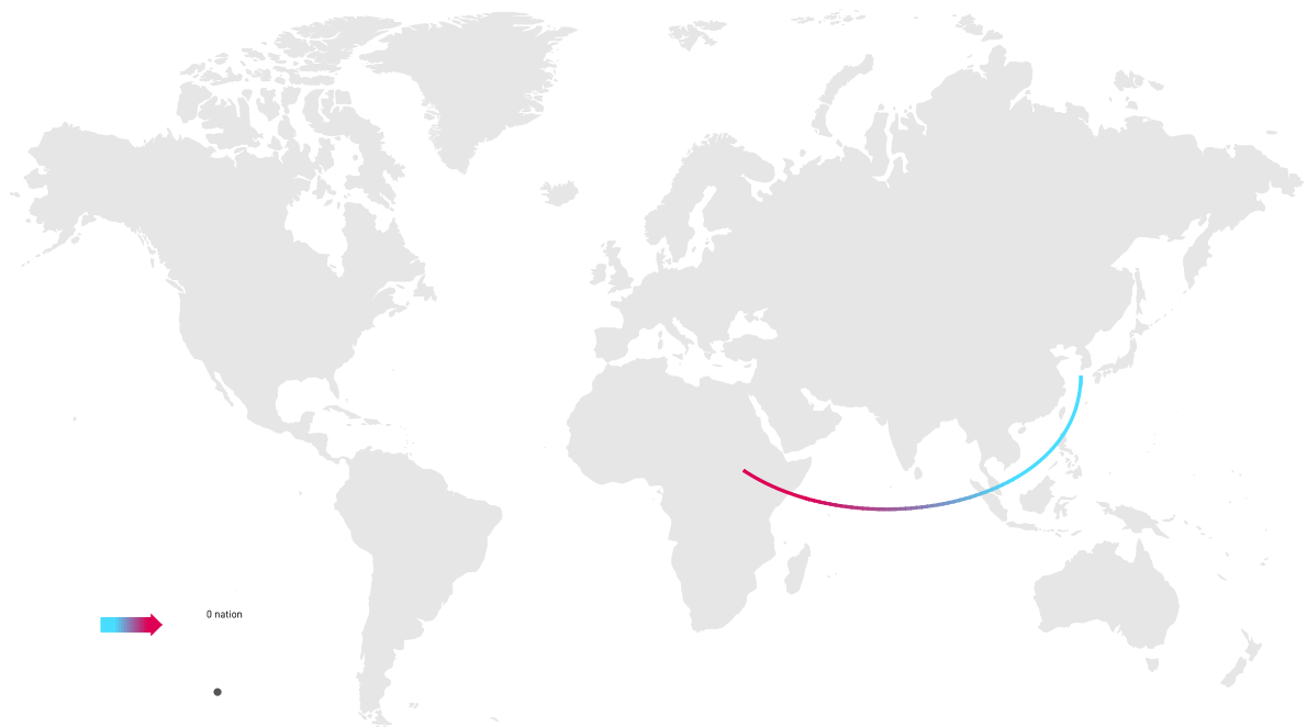
図 1 : G20 各国の消費により発生する PM 2.5 に由来する乳幼児（5 歳未満）早期死亡数 ; 消費国と影響国 ("to") のネットワーク関係
