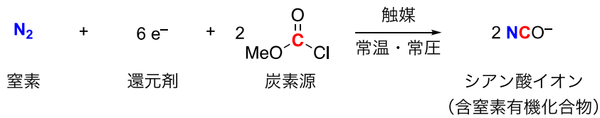
図2 窒素ガスから直接、触媒的に含窒素有機化合物を合成する手法
