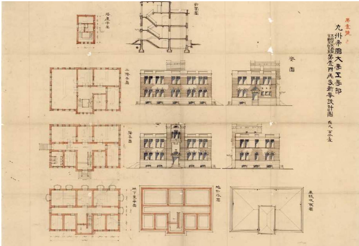
資料9 大正13年 「九州帝国大学工学部本館焼失為仮実験室研究室第一附属家新築設計図」より姿図及び各階平面図 【九州大学大学文書館所蔵】 本部建築課棟。工学部本館が完成する以前は、仮実験室として使用されていた。
