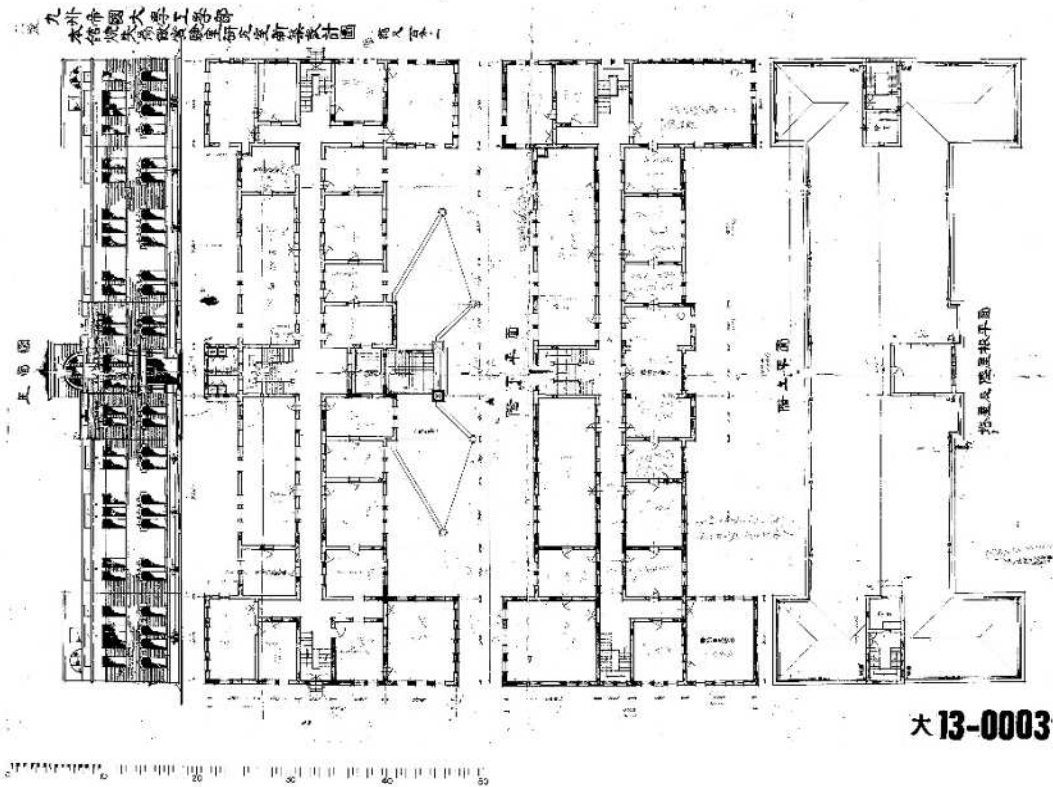
資料6 大正13年 「九州帝国大学工学部本館焼失為仮実験室研究室新築設計図」より各階平面図 【九州大学大学文書館所蔵】 本部事務室棟。工学部本館が完成する以前は、仮実験室及び研究室等として使用されていた。
