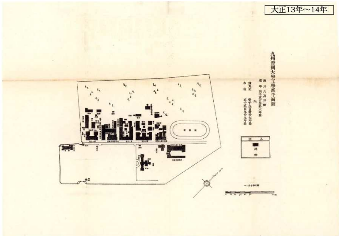
資料12 大正13~14年 九州帝国大学工学部平面図 【九州大学大学文書館所蔵】 法文学部本部・法文学部図書館及び書庫の建設のためキャンパスが拡大された。 正門位置の変更に伴い、門衛所は曳家によって正門内側右手に移築された。 前年度の図と比較すると、工科大学本館が描かれておらず、火災により焼失してしまったことがわかる。
