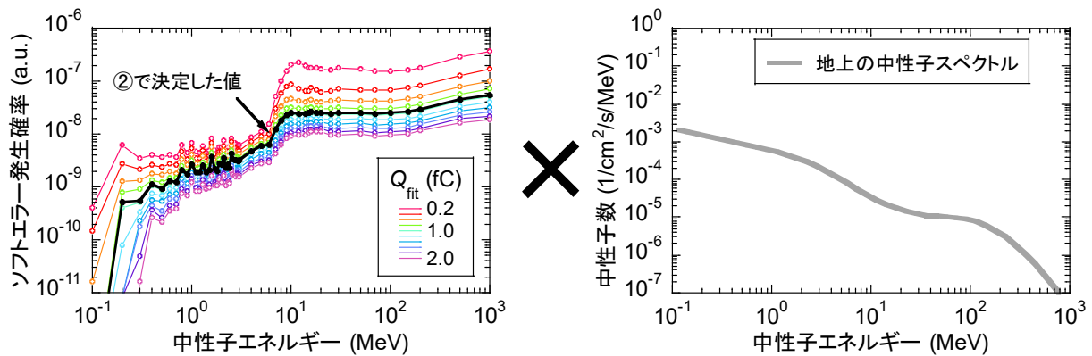
図 1. 地上環境のソフトウェア率の見積もり手順
