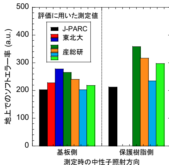
図3 各測定値を用いたソフトエラー率の見積結果
