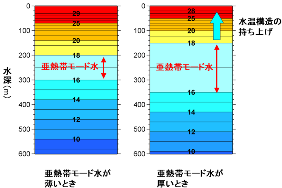
図 2：亜熱帯モード水による「持ち上げ効果」の模式図
