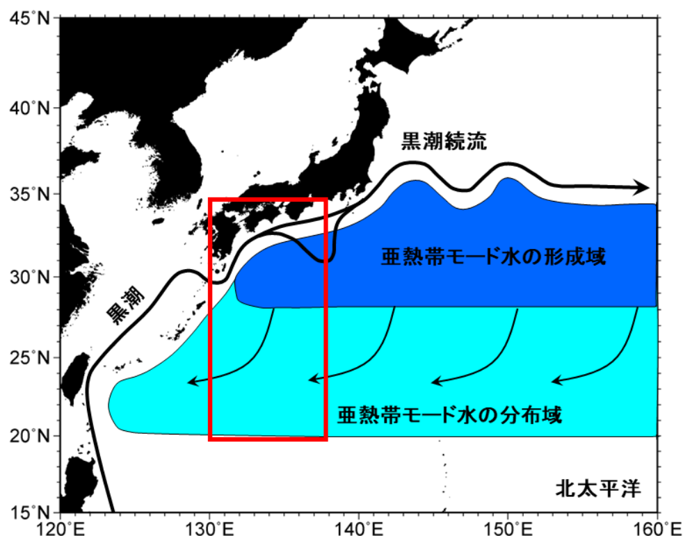
図 3：亜熱帯モード水の形成域（青）と分布域（水色）の分布
