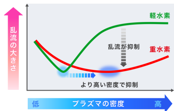
図3 軽水素プラズマと重水素プラズマでの乱流のふるまいの違い
