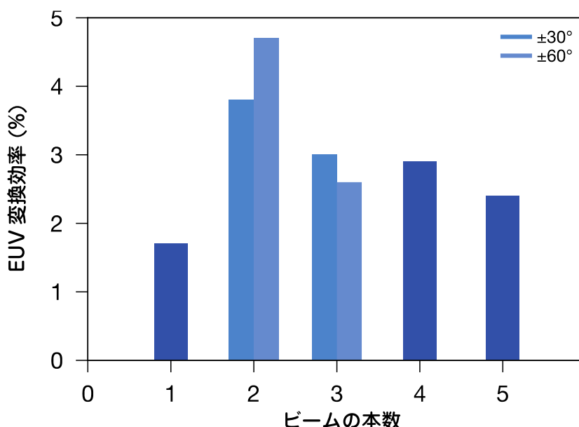
図 2 : EUV 変換効率のレーザ照射ビーム数依存性。ビームが 2 本のときの EUV 変換効率が最も大きくなりました。時間的に同期した 2 台の独立レーザを用意し、同時にレーザパルスを照射することで EUV 変換効率を 2 倍以上に増加させることができました。このことは、1 台あたりのレーザシステムの出力を下げてもよいことを意味しています。レーザシステムの高出力化に伴い開発負荷を下げられる上、EUV 変換効率も向上することから、低消費電力化あるいは EUV 光源の高出力化につながることを示しています。
