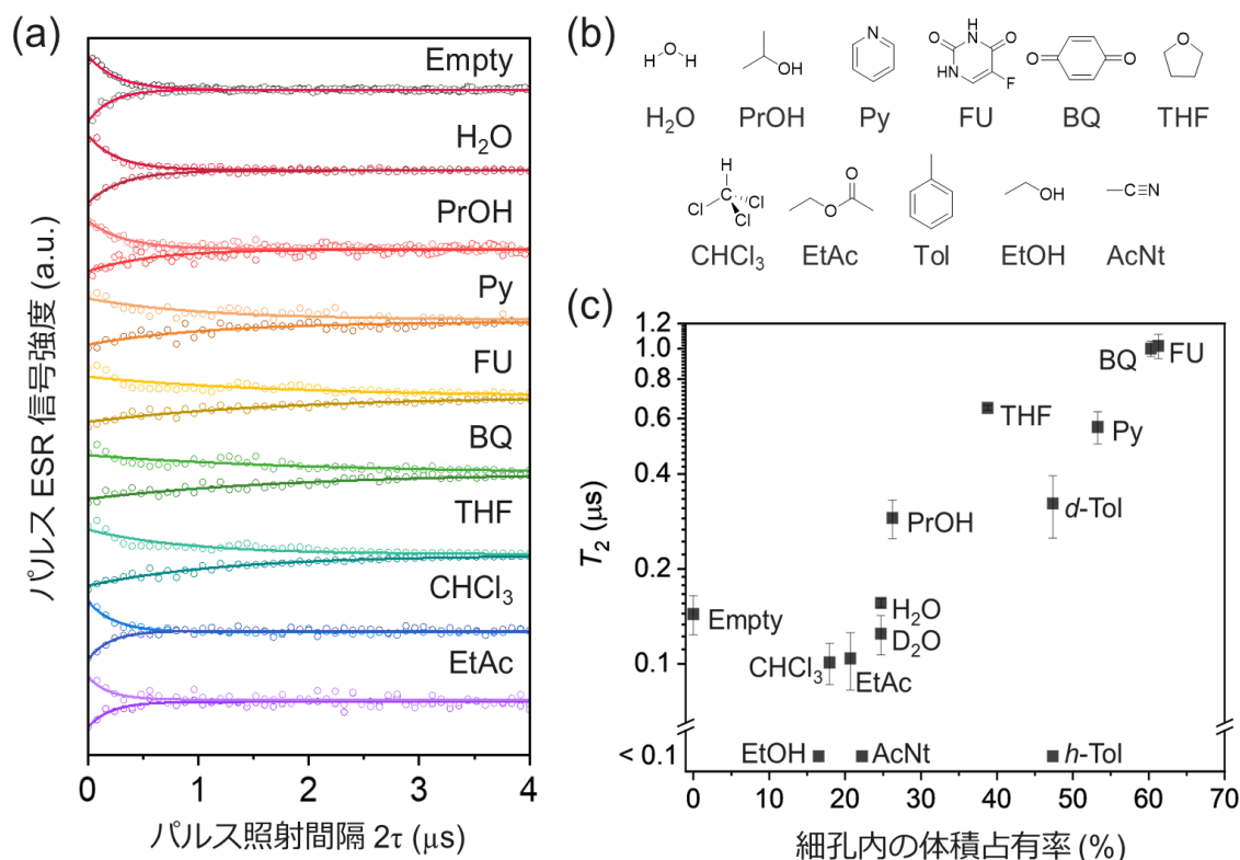
図 2 (a) 各ゲストを導入した際の T_2 測定結果。MOF 中に量子ビット以外の分子が存在しない空の状態 (Empty) に比べ、ゲストの導入によって T_2 が長くなる挙動が見られた。
