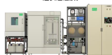
図2 減圧蒸気スweep型のCO 2 膜分離装置モデル図。
