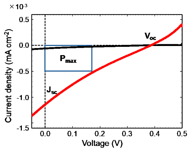
(図3) 有機熱電デバイスの J-V 特性。赤線が CuPc(180 nm)/F 16 CuPc(320 nm)/C 60 (20 nm)/BCP(20 nm)の素子特性。 V OC : 開放端電圧、J SC : 短絡電流、P max : 最大電力。
