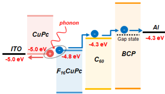
(図1) 新型有機熱電デバイスの動作機構 (エネルギー準位と電荷の移動の様子)。
