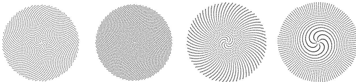
図 2 左から順に黄金比の次、その次に高いパッキング密度となる白銀比 1 + \sqrt{2} と (9 + \sqrt{221})/10 の場合（密度 \gtrsim \pi/4\sqrt{2} \doteq 0.555 , \gtrsim 5\pi/2\sqrt{221} \doteq 0.528 ）、 \pi , e を用いた場合のフォーゲル螺旋。
