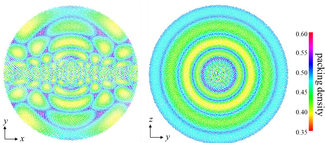
図 4 3次元球体における点群生成。断面図を示す。パッキング密度で点群を着色。
