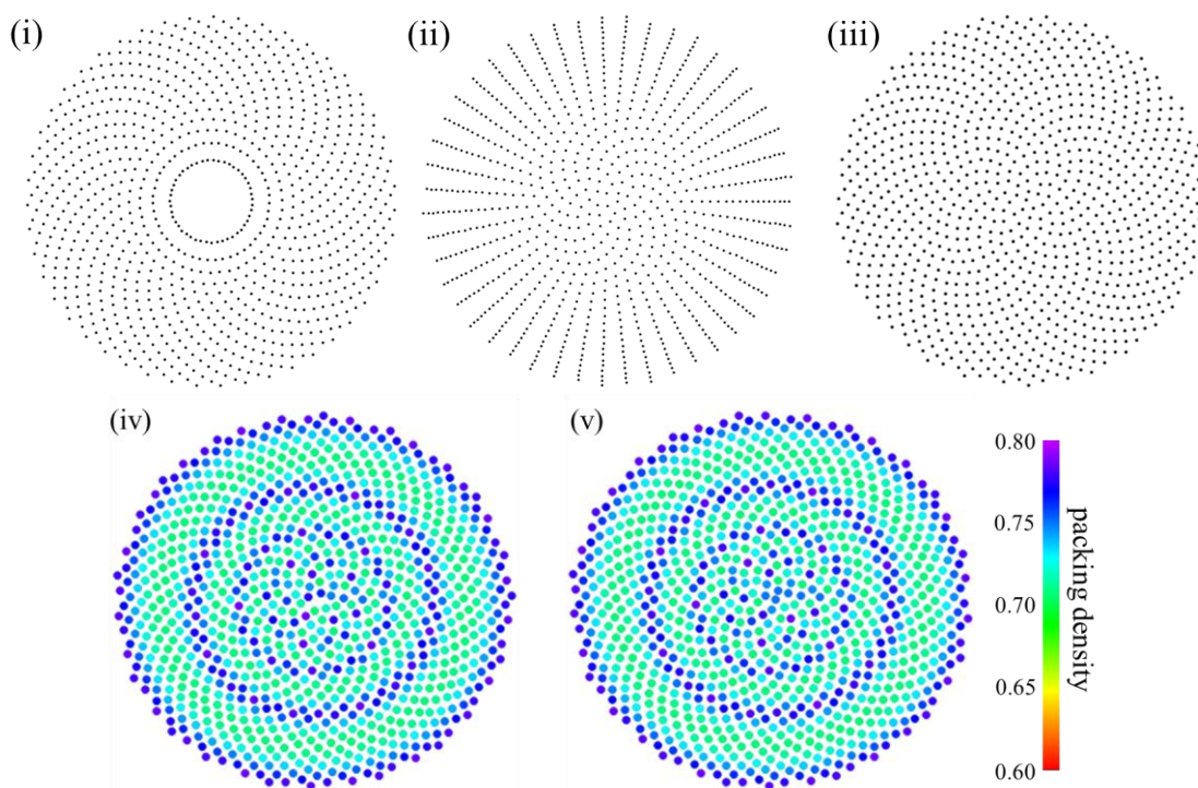
図 3 (i), (ii), (iv)は既存手法、(iii), (v)は提案手法による。フォーゲル螺旋では中心点付近を除きほとんど同じだが、他の写像を用いると(i)―(ii)のように均一にならないことが一般化の障害であった。パッキング密度で点群を着色。
