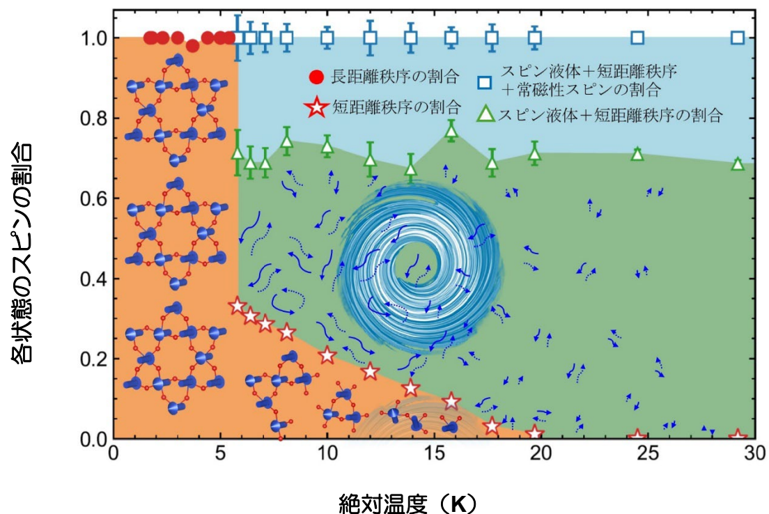
図 2. スピン液体（青い矢印ペア）とせめぎ合いながら、線形的に成長するスピ ンクラスター（短距離秩序）（白抜き赤★）の様子。5.5K の温度でスピ ンクラスターの割合がスピン液体と等しくなり、すべてのスピが一気につな がった長距離秩序（塗りつぶし赤●）へ転移する。
