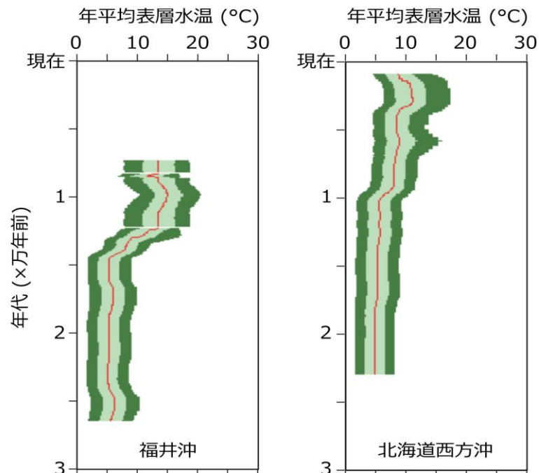
参考図 3. (左) 福井沖および (右) 北海道西方沖における過去 2 万年間の水温復元結果 (表層水の年平均水温)
