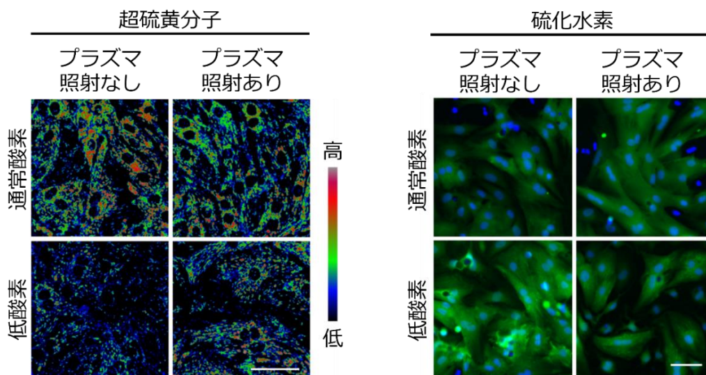
図 2 システインプラズマ照射が硫黄代謝に与える効果
