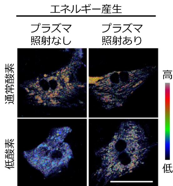
図 1 システインプラズマ照射はミトコンドリアでのエネルギー産生を回復させる
