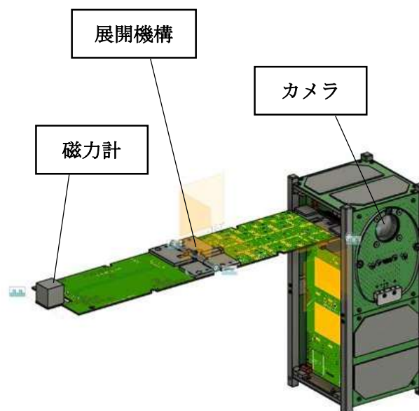
展開機構展開図
