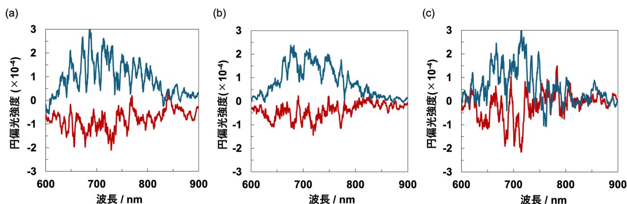
図3 (a)CzTTBrM、(b)2CzTTBrM、(c)3CzTTBrM の円偏光発光(CPL)スペクトル
