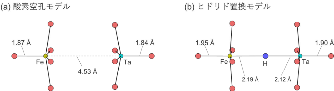
図 2. (a) 酸素空孔と (b) ヒドリド置換における局所構造を比較しています。酸素空孔モデルではタンタル近傍で結合バランスが崩れ大きな歪みが生じるのに対し、ヒドリド置換モデルではヒドリドの導入により歪みが緩和され、より安定な構造が得られています。
