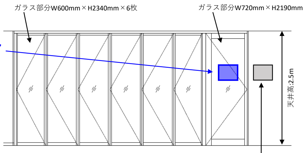
②ミーティングラウンジ側展開図
