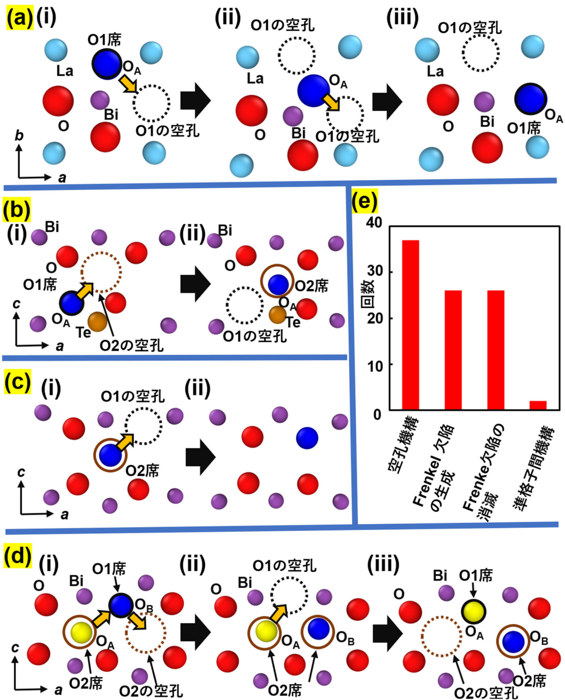
図4 本研究で発見した \text{Bi}_{1.9}\text{Te}_{0.1}\text{LaO}_{4.05}\text{Br} における (a) 空孔機構による酸化物イオンの高速拡散のスナップショット。(b) Frenkel 欠陥 (用語 11) の生成過程。(c) Frenkel 欠陥の消滅過程。(d) 準格子間機構による酸化物イオンの高速拡散のスナップショット。(e) 各イベントの回数のヒストグラム：準格子間機構に比べて、空孔機構による移動の回数が極めて多い。このことは酸化物イオンの長距離拡散が主として空孔機構により生じていることを示している。©論文の著者 (2026)
